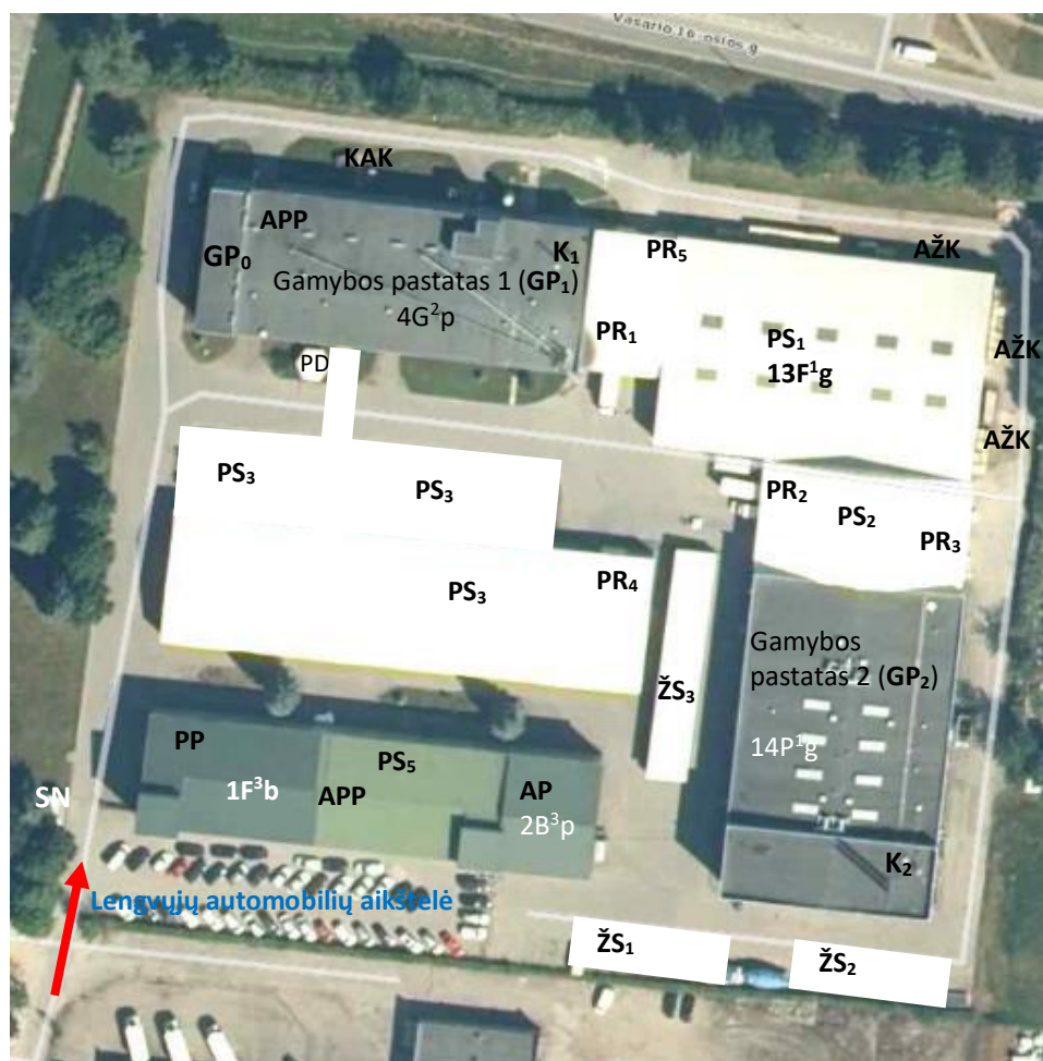
Pav. 2. UAB „BEWI Lithuania“ administracijos, gamybos ir sandėliavimo zonų išdėstymo žemės sklype planas
