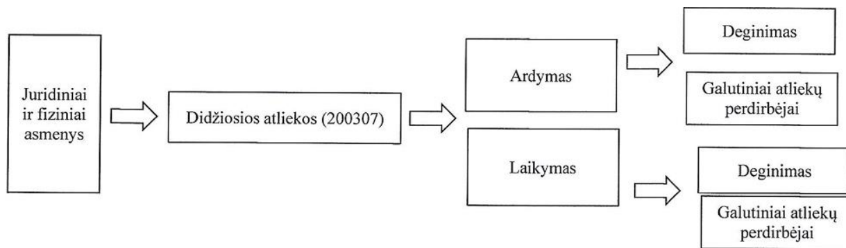
Pav. 3. Didelių gabaritų atliekų tvarkymo technologinio proceso schema
