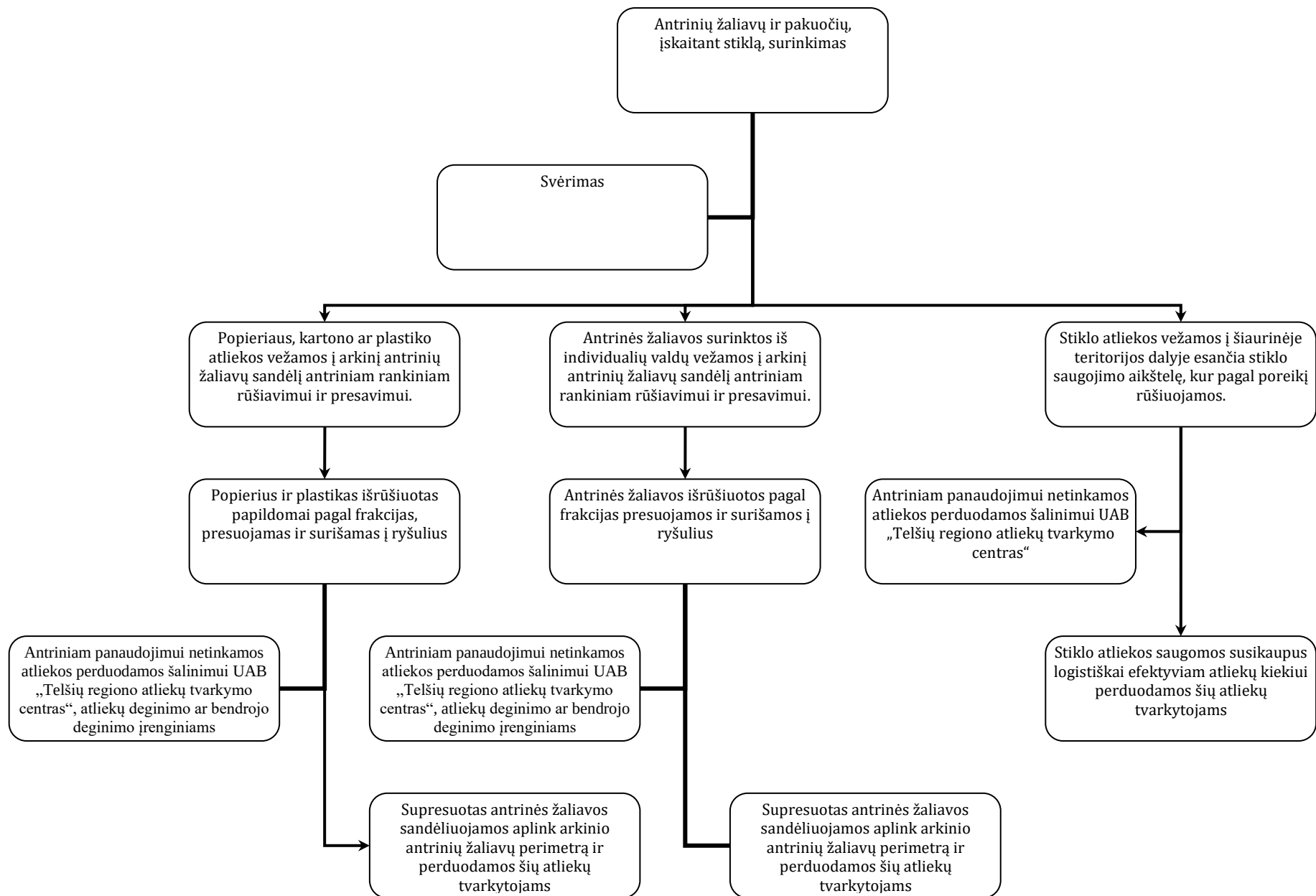
Pav. 2. Antrinių žaliavų, įskaitant stiklą, tvarkymo technologinė schema
