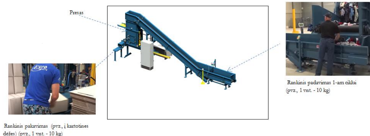
Pav. 6 Pusiau automatinės presavimo / pakavimo rūšiavimo linijos Z10R AV-TVS pavyzdys (1 ciklas - 20 sek.; 180 vnt. x 10 kg / val.; 1,8 t/val.) https://www.youtube.com/watch?v=9pcOJBHSto&feature=youtu.be
